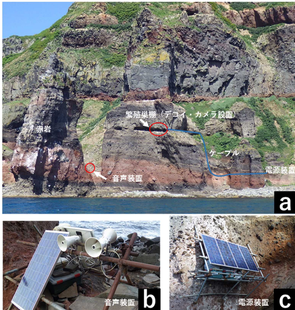
図 1. (a) 赤岩の対岸に位置するウミガラスの繁殖巣棚 (赤岩対崖) と全体の概要. (b) 音声装置の概要. 音声装置は、2 枚の太陽電池パネルで 1 つのバッテリーを充電して、4 つのスピーカーからウミガラス声を日中のみ再生した. (c) 電源装置の概要. 電源装置は 4 枚の太陽電池パネルで 4 つのバッテリーを充電した. 約 60m のケーブルで繁殖地に設置した CCD カメラに電力供給し、太陽電池パネルの下に設置した録画装置に映像を記録.
