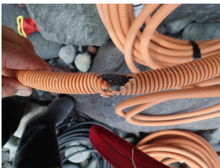
図 3. ケーブルの損傷状況
