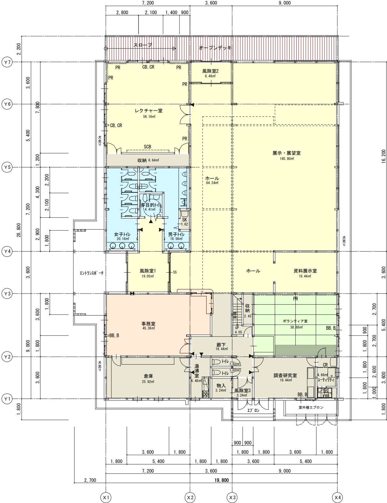
1 F 平面図
