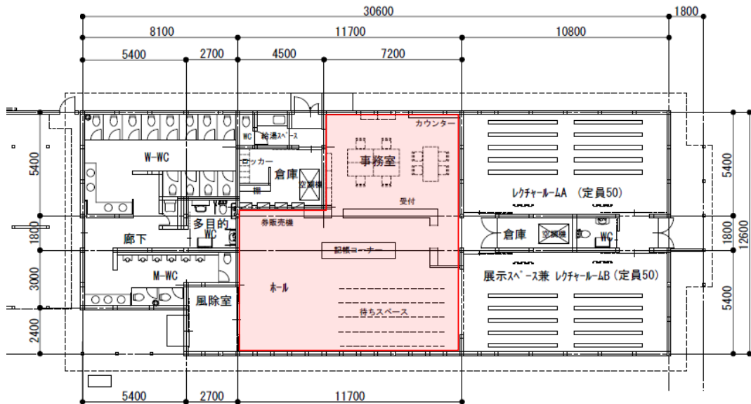
フィールドハウス平面図
