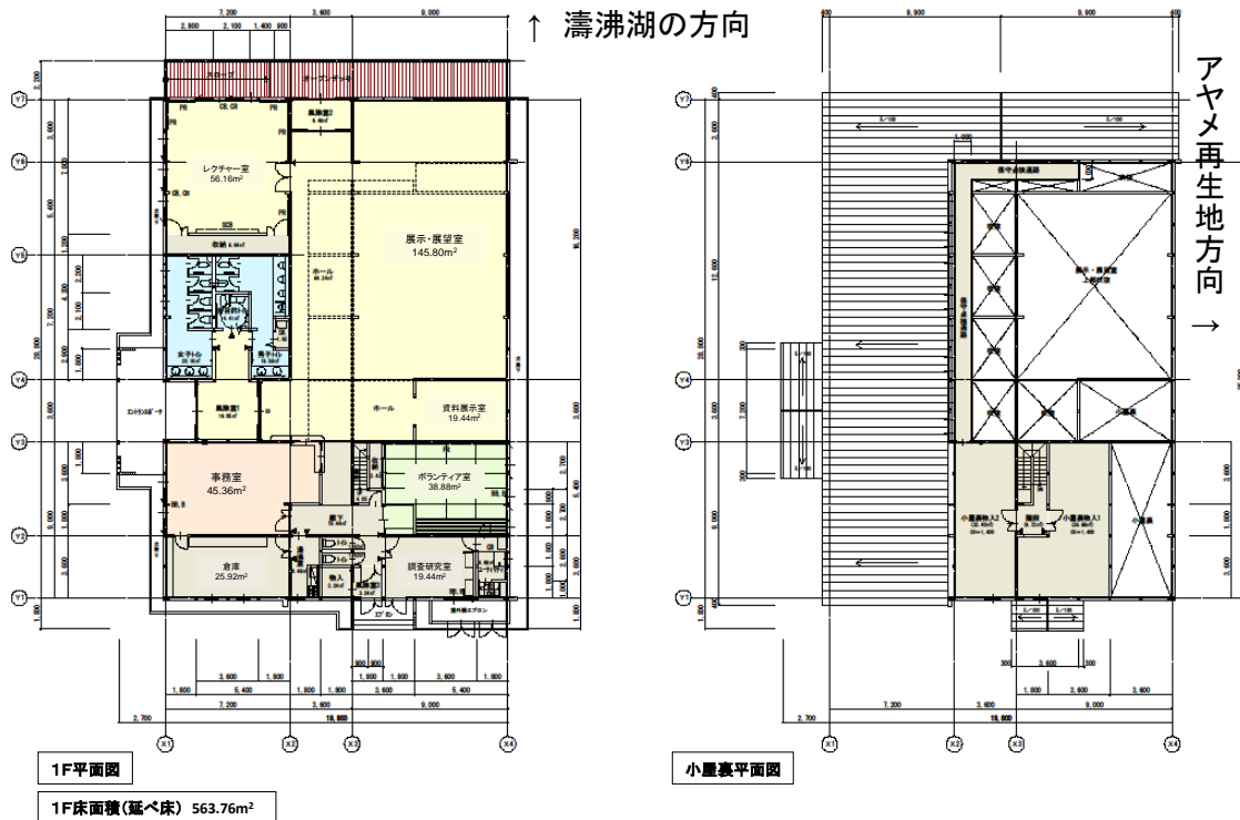
建物平面図(変更後)
