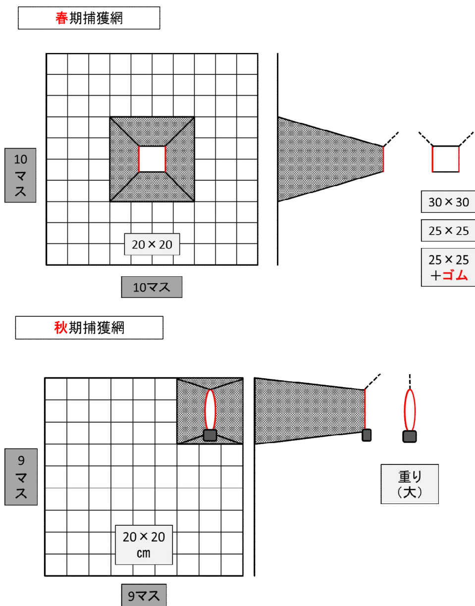
図7. 定置網に設置した漏斗式捕獲網の構造（春期、秋期）
