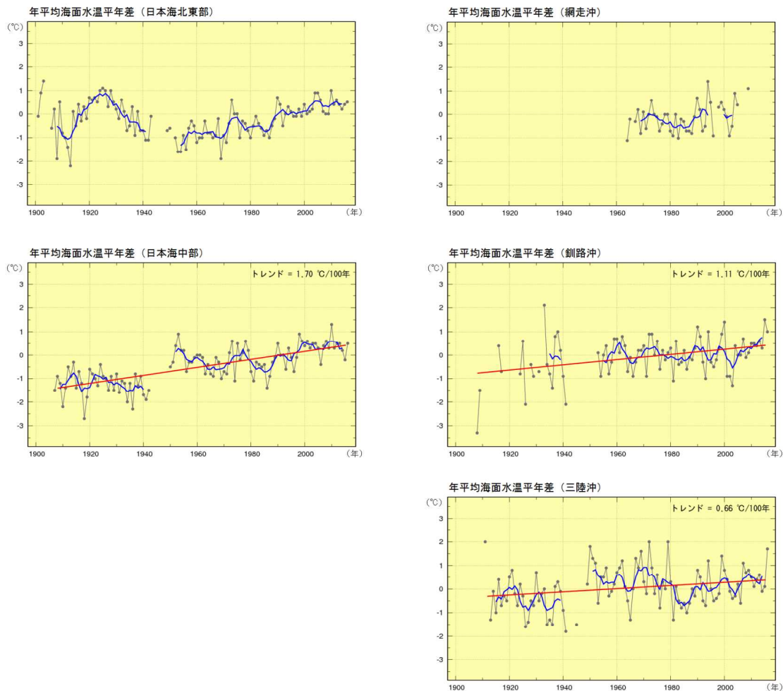
図4-6 各海域における年平均海面水温の経年変化 (単位: °C)
