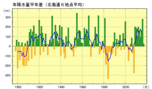
図4-3 北海道6地点（旭川、網走、札幌、帯広、根室、寿都）を平均した年降水量の経年変化（1898～2017年、単位：mm） 棒グラフは各観測地点での年降水量の基準値からの偏差を平均した値を示している。青線は偏差の5年移動平均を示す。基準値は1981～2010年の30年平均値。
