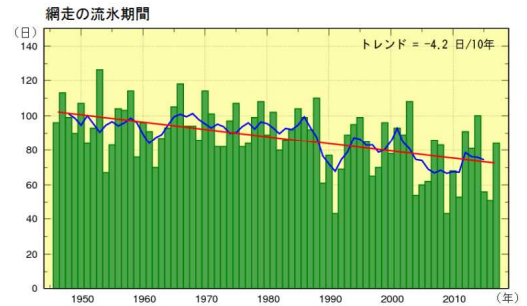
図4-7 網走における流氷期間の経年変化 (1946～2017年、単位：日)
