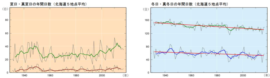
図4-2 北海道5地点（網走、札幌、帯広、根室、寿都）で平均した夏日、真夏日、冬日、真冬日の1地点あたり年間日数の経年変化（1931～2017年、単位：日） 左図は夏日（緑）、真夏日（茶）の経年変化を、右図は冬日（緑）および真冬日（青）の経年変化をそれぞれ示す。細線は各年の値を、太線は5年移動平均をそれぞれ示し、直線（赤）は期間にわたる変化傾向を示す。なお、真夏日の日数は夏日の日数に、真冬日の日数は冬日の日数にそれぞれ含まれる。
