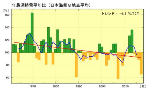
図4-4 北海道日本海側8地点（稚内、留萌、旭川、札幌、岩見沢、寿都、江差、倶知安）を平均した年最深積雪年比の経年変化（1962～2017年、単位：%） 観測点ごとに年最深積雪の1981～2010年平均に対する比を求め、地域内の全地点を平均した値を示している。青線は偏差の5年移動平均を、赤線は期間にわたる変化傾向を示している。なお、棒グラフは比の基準値（100%）からの差を示し、緑（黄色）の棒グラフは基準値から増えている（減っている）ことを示している。
