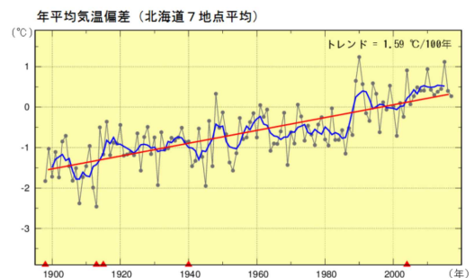
図4-1 北海道7地点（旭川、網走、札幌、帯広、根室、寿都、函館）を平均した年平均気温の経年変化（1898～2017年、単位：℃）
