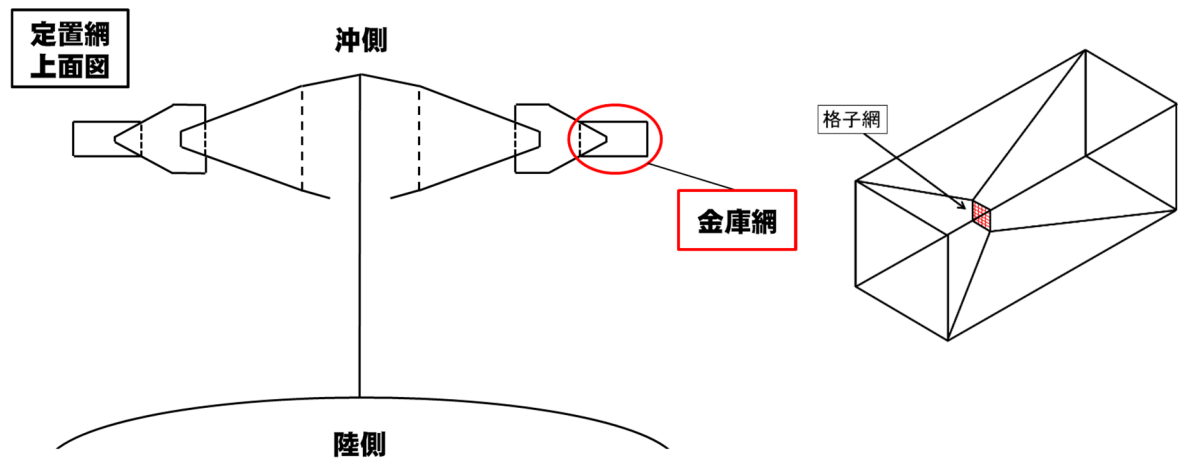
図1. 防除用格子網の設置状況
