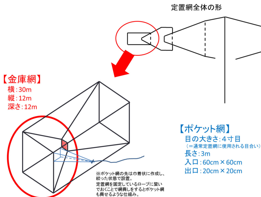
図9. ポケット網構造
