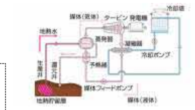
一般的なバイナリー発電システム構成図
