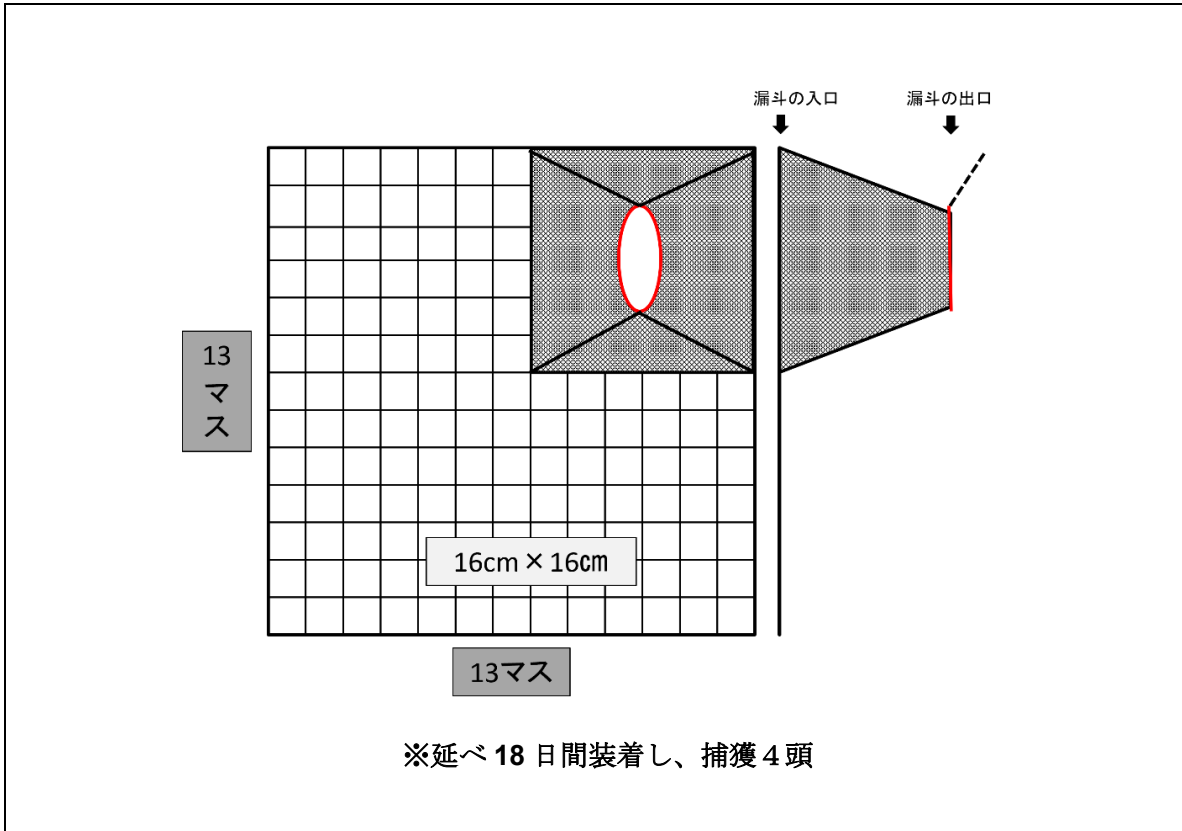
図 12. B 定置網で使した捕獲網（漏斗の入口：縦5目×横5目）
