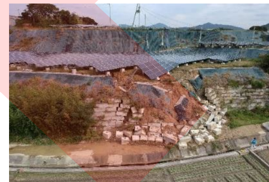
法面保護工が崩れて流出した事例
