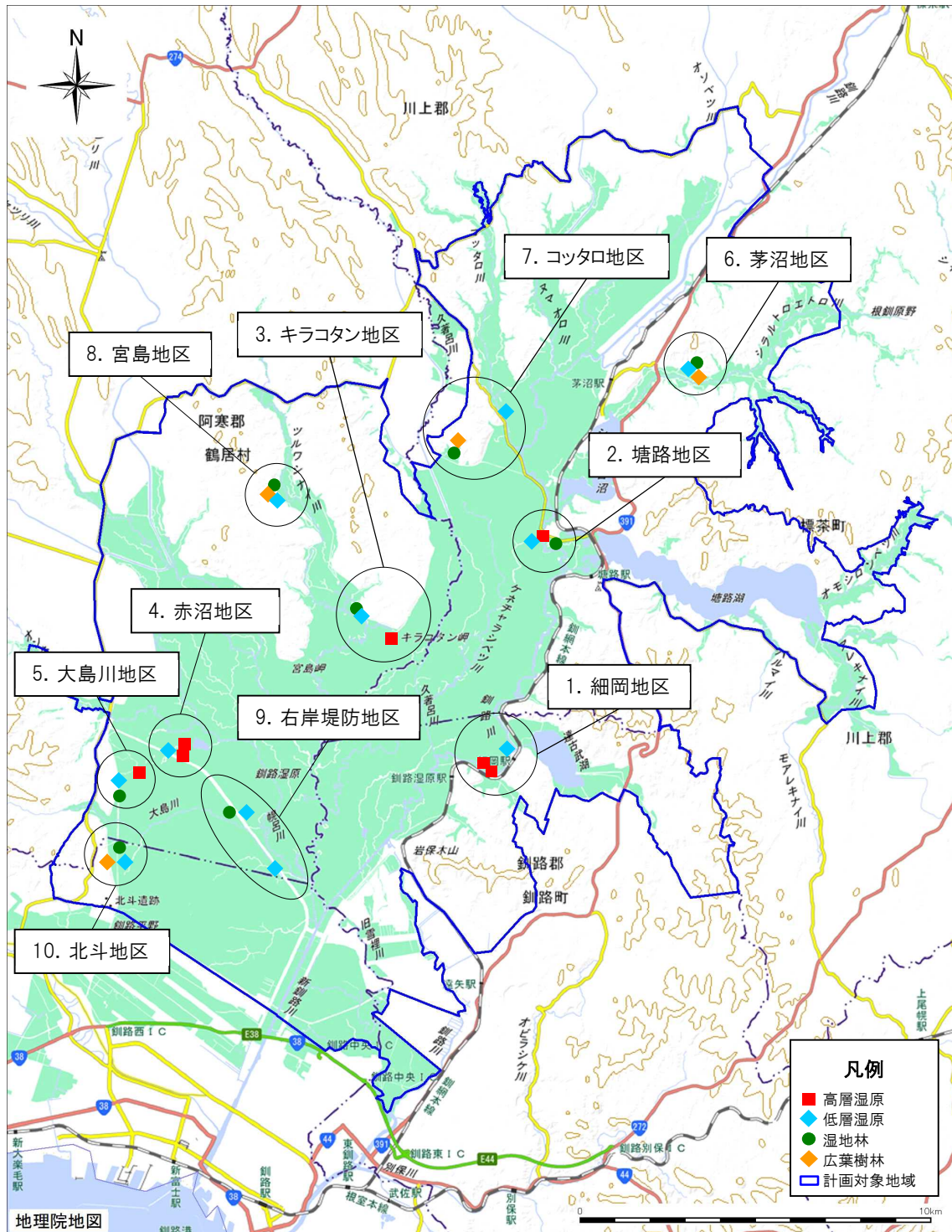
図 4. 植生調査実施位置図
