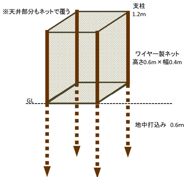
図2 簡易植生保護柵の構造例
