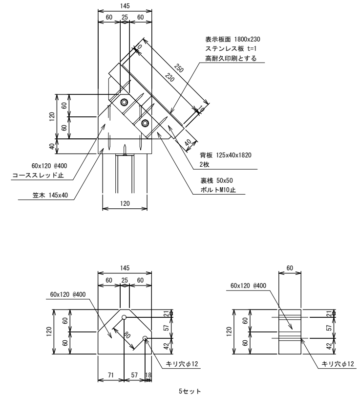
断面詳細図
