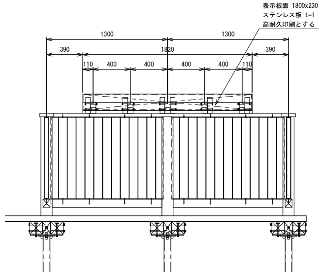
正面図
