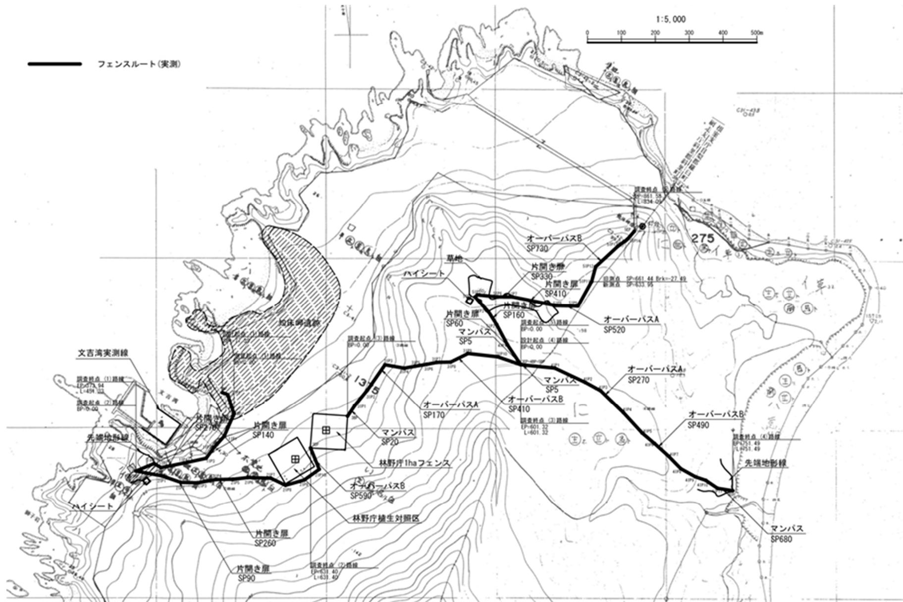
図 1. 知床岬地区仕切柵既設位置図
