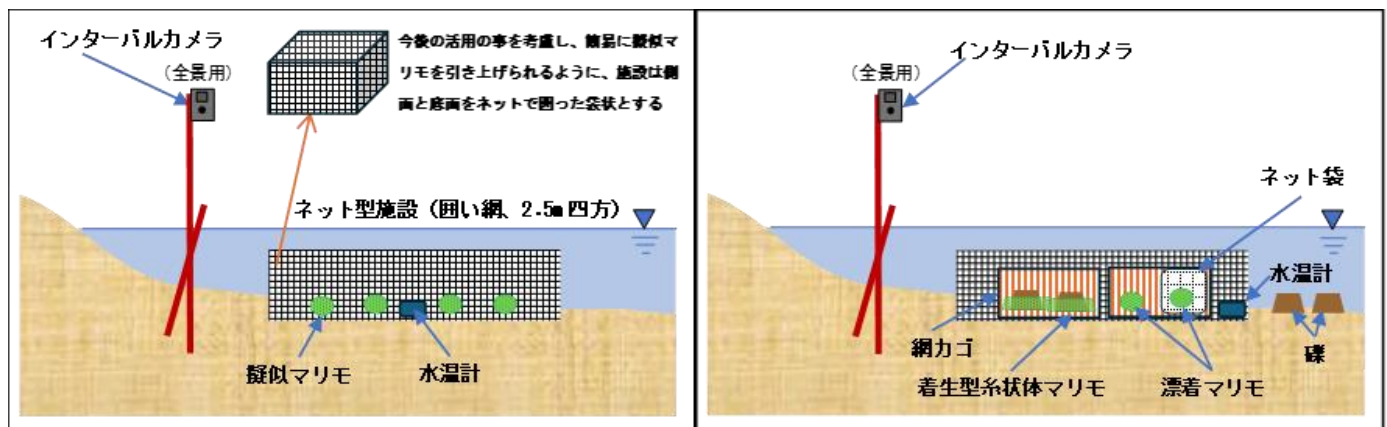
図3 ネット型施設概略
